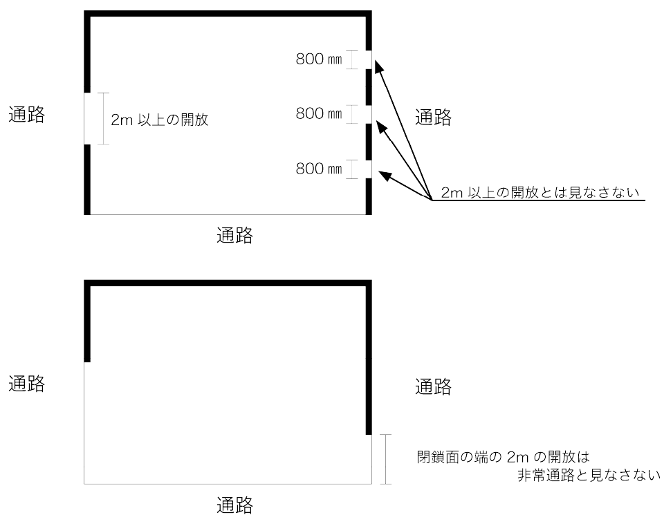
図8 100m 2 以上の小間の開放面について
